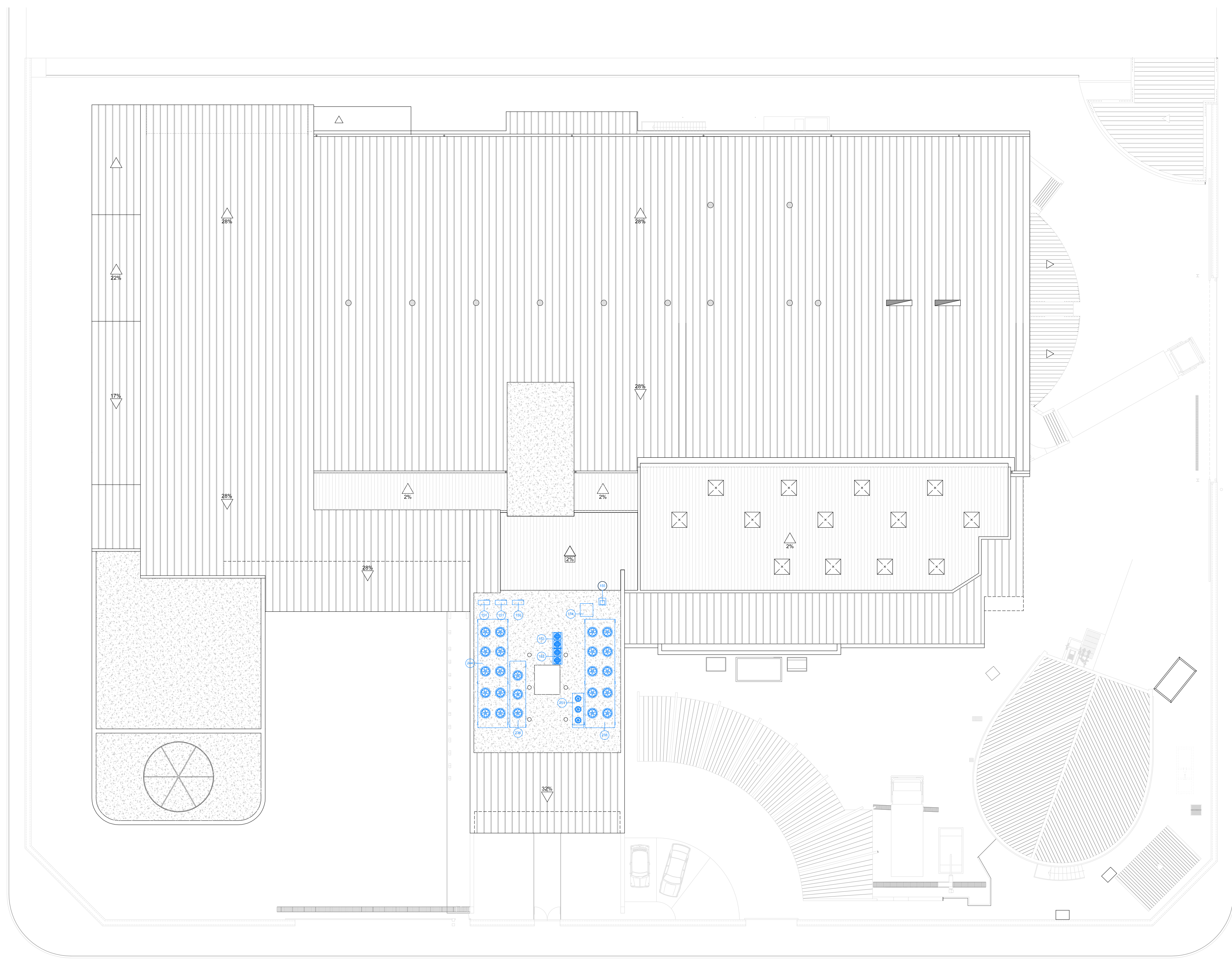
PLANTA COBERTA E: 1/200
